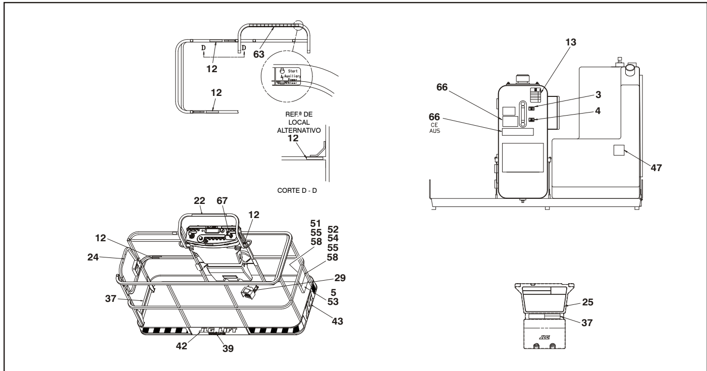
Figura 4-13. Instalação dos autocolantes 600A e 600AJ - Página 3 de 4
