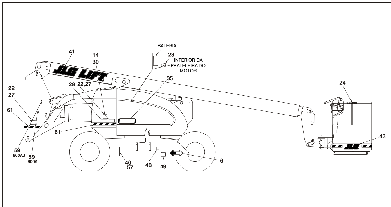
Figura 4-12. Instalação dos autocolantes 600A e 600AJ - Página 2 de 4
