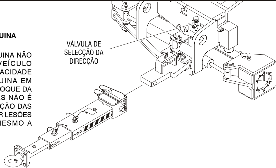
Figura 4-7. Pontos de fixação da barra de reboque - de S/N 81836 à actualidade
