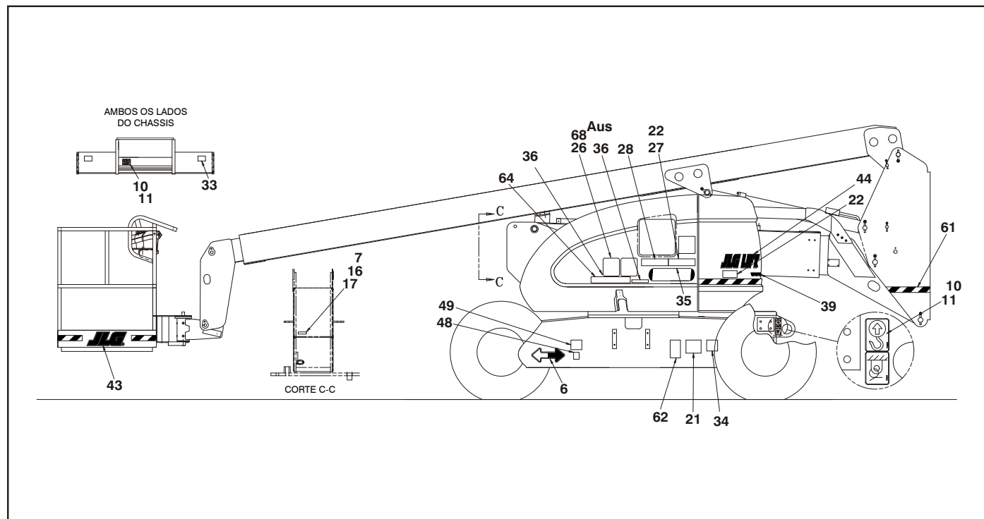
Figura 4-11. Instalação dos autocolantes 600A e 600AJ - Página 1 de 4
